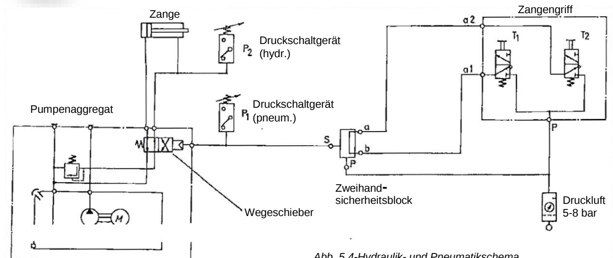
Abb. 5.4-Hydraulik- und Pneumatikschema
