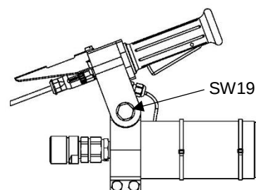
Abb. 5.8 Griffhalter
