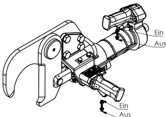
Abb. 6.1 – Handgriffe mit Schalter
