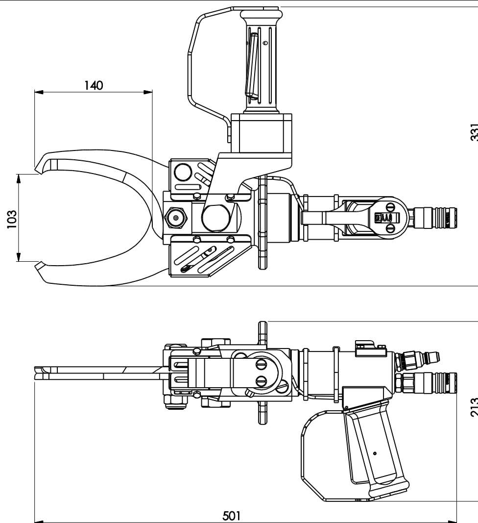
Maßskizze
