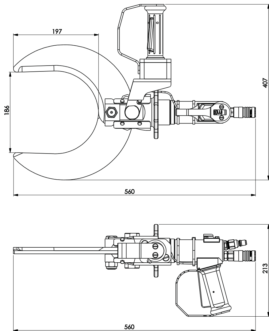
Maßskizze
