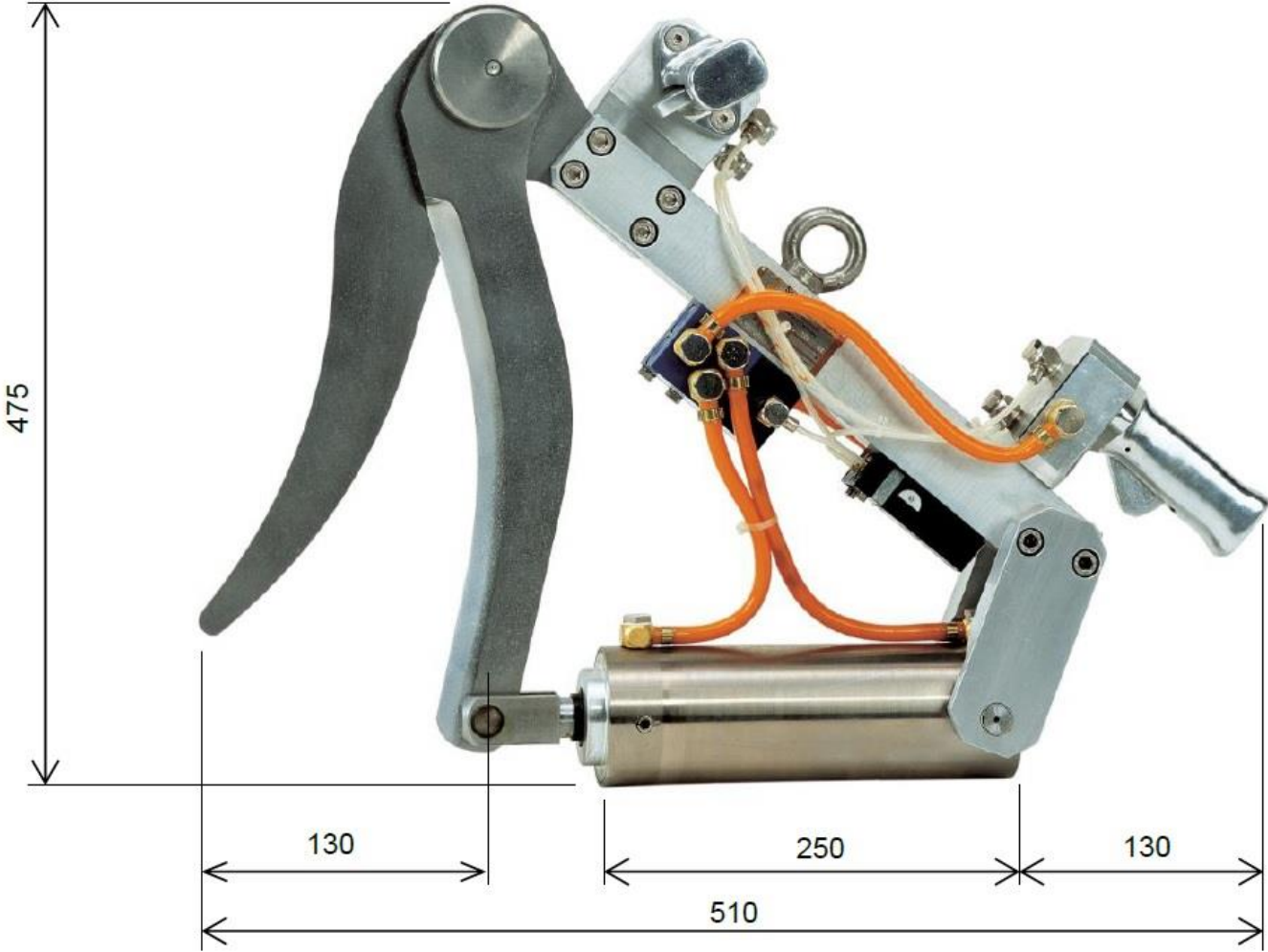
Maßskizze
