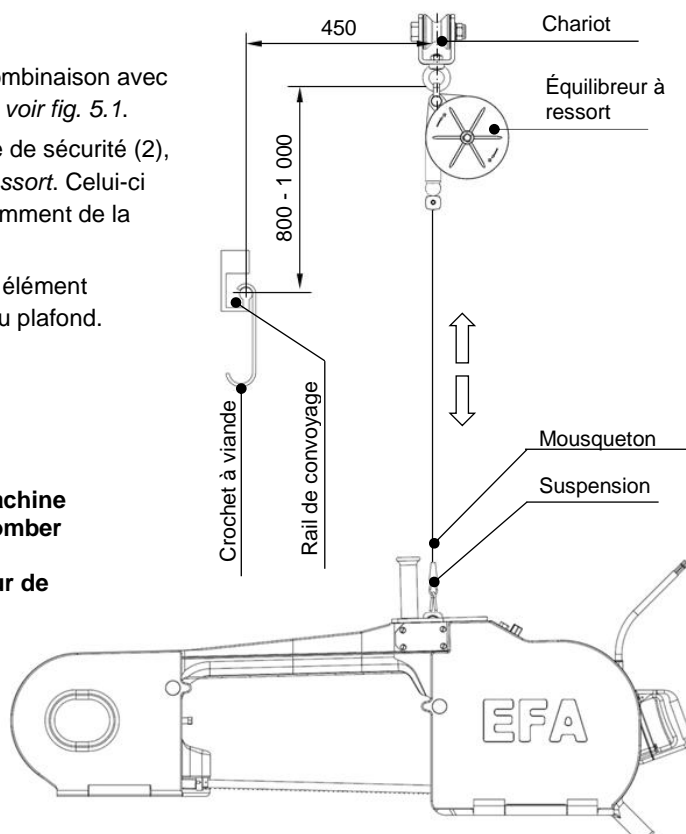
Fig. 5.1 – Système réducteur de poids (équilibreur à ressort)
