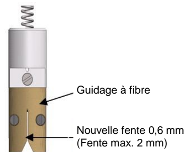
Fig. 7.3 – Remplacement du guidage
