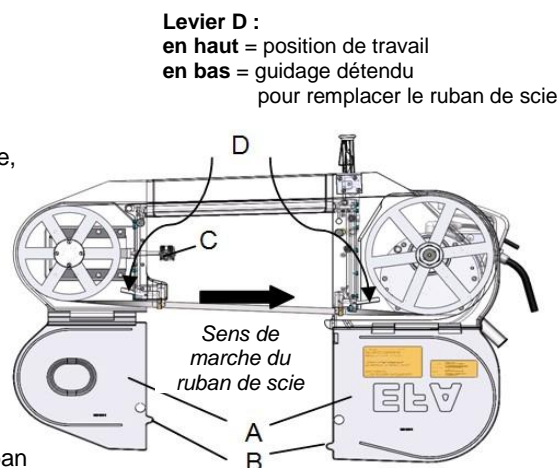
Fig. 7.1 – Remplacement du ruban de scie
