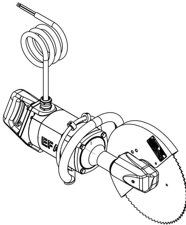
Zerlegesäge EFA 85
